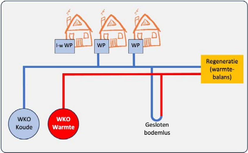
figuur 1: schema ZLT warmtenet
