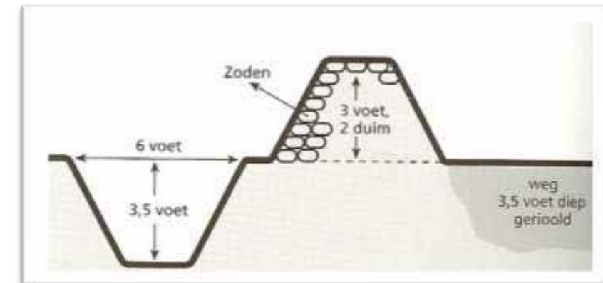
Afbeelding 1: Doorsnede van een houtwal.
